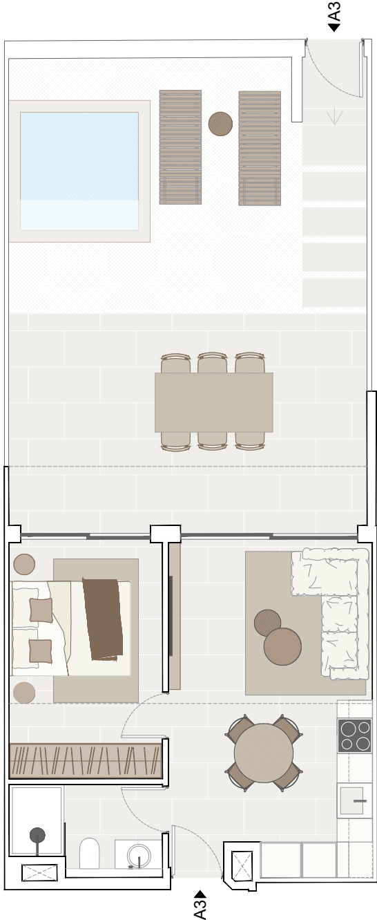
Vivienda A3. E = 1/30
