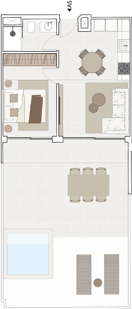
Vivienda A5. E = 1/30
