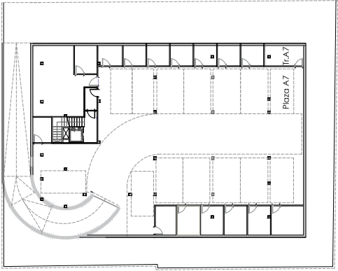
Planta sótano. E = 1/200 Ubicación de la plaza de aparcamiento y del trasero
