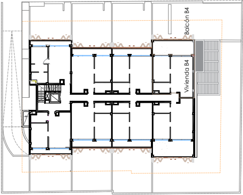
Planta primera. E = 1/200 Ubicación de la vivienda
