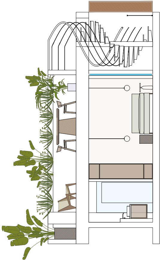
Sección 1 Vivienda B4. E = 1/30
