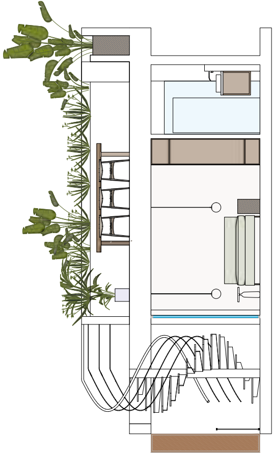
Sección 1 Vivienda B5, E = 1/30
